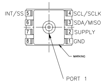
MS4515DO-TPvoixxyP
